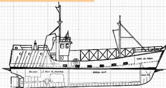
PERFIL
